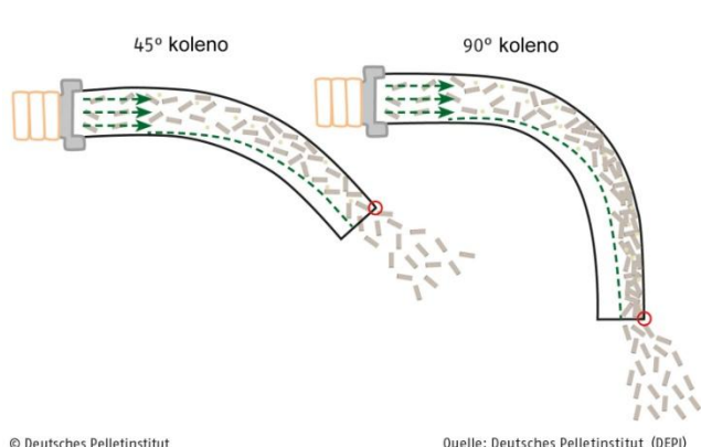
Obrázek 8: Modely foukání pelet skrze různé ohyby bez použití vhodného rovného stabilizačního dílu
